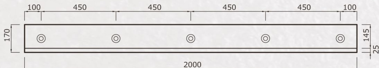
正面図
