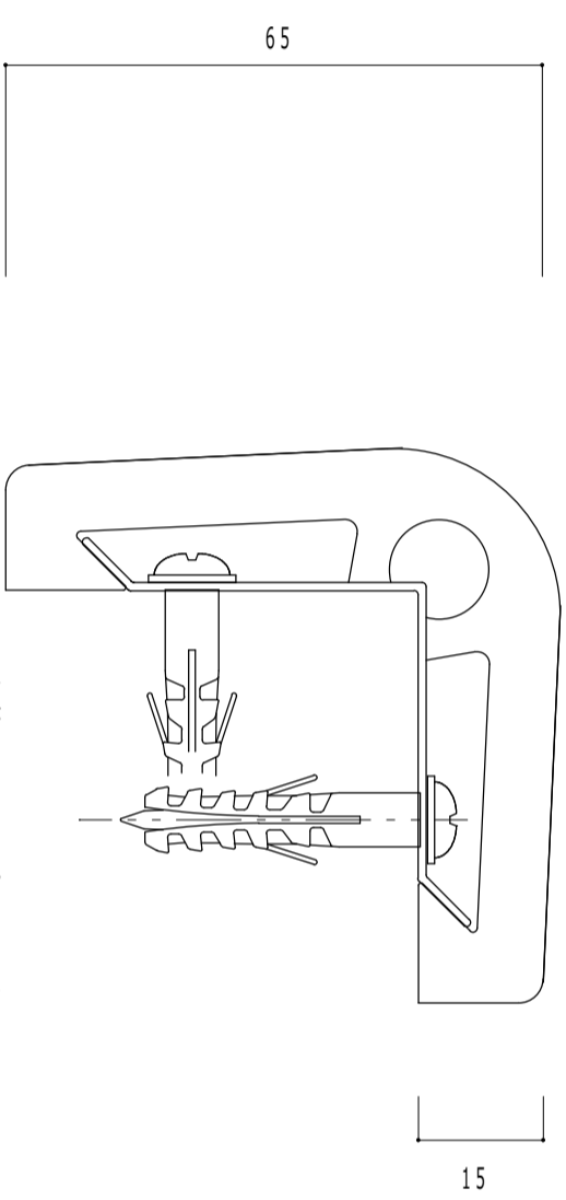
本体+ベースプレート断面図
