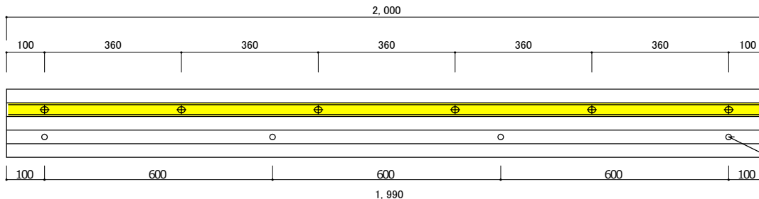
□ 本体正面図
